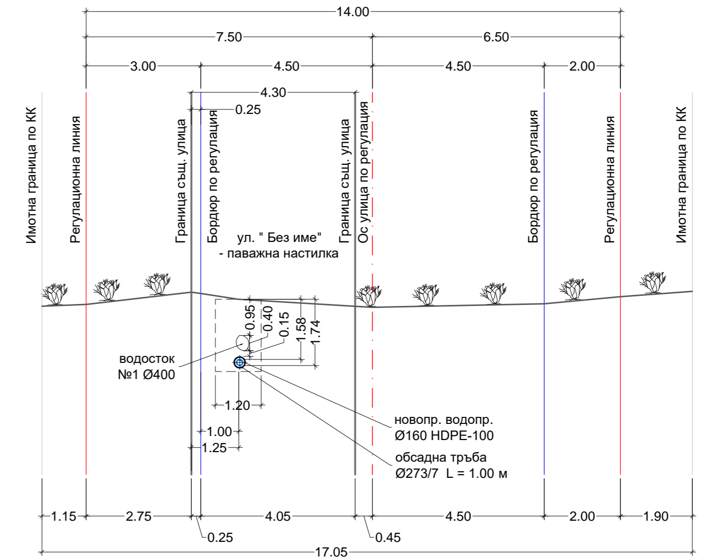
НАПРЕЧЕН РАЗРЕЗ №8 - хоризонтално сондиране
