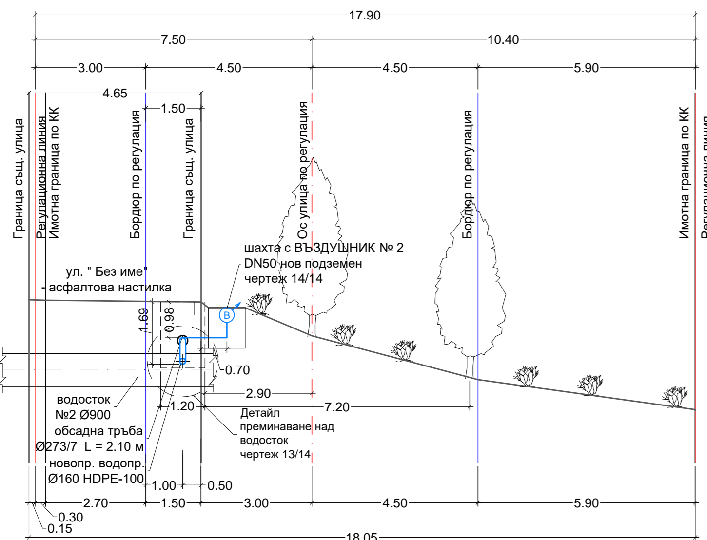
НАПРЕЧЕН РАЗРЕЗ №9 - открит вертикален изкоп
