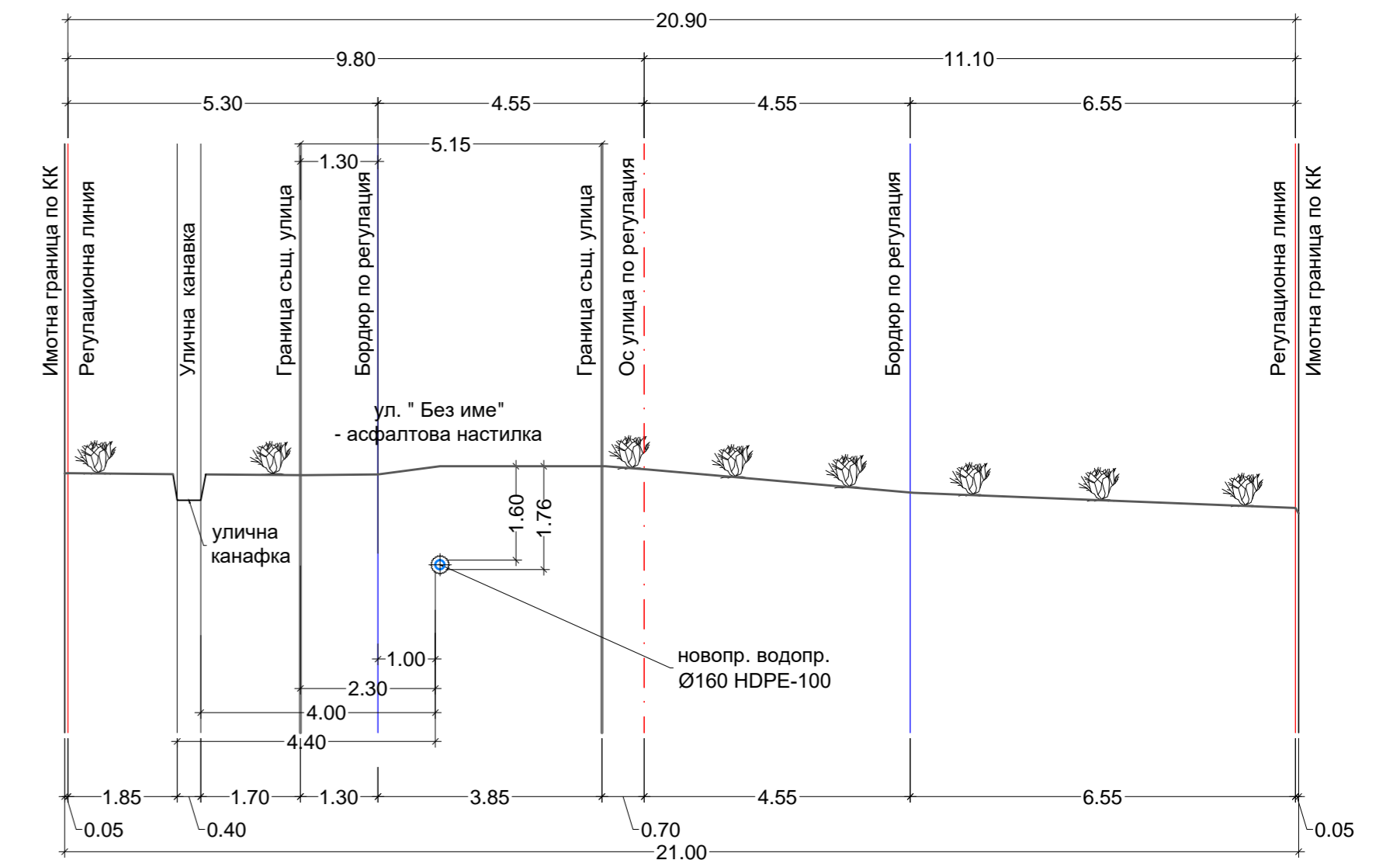
НАПРЕЧЕН РАЗРЕЗ №12 - хоризонтално сондиране
