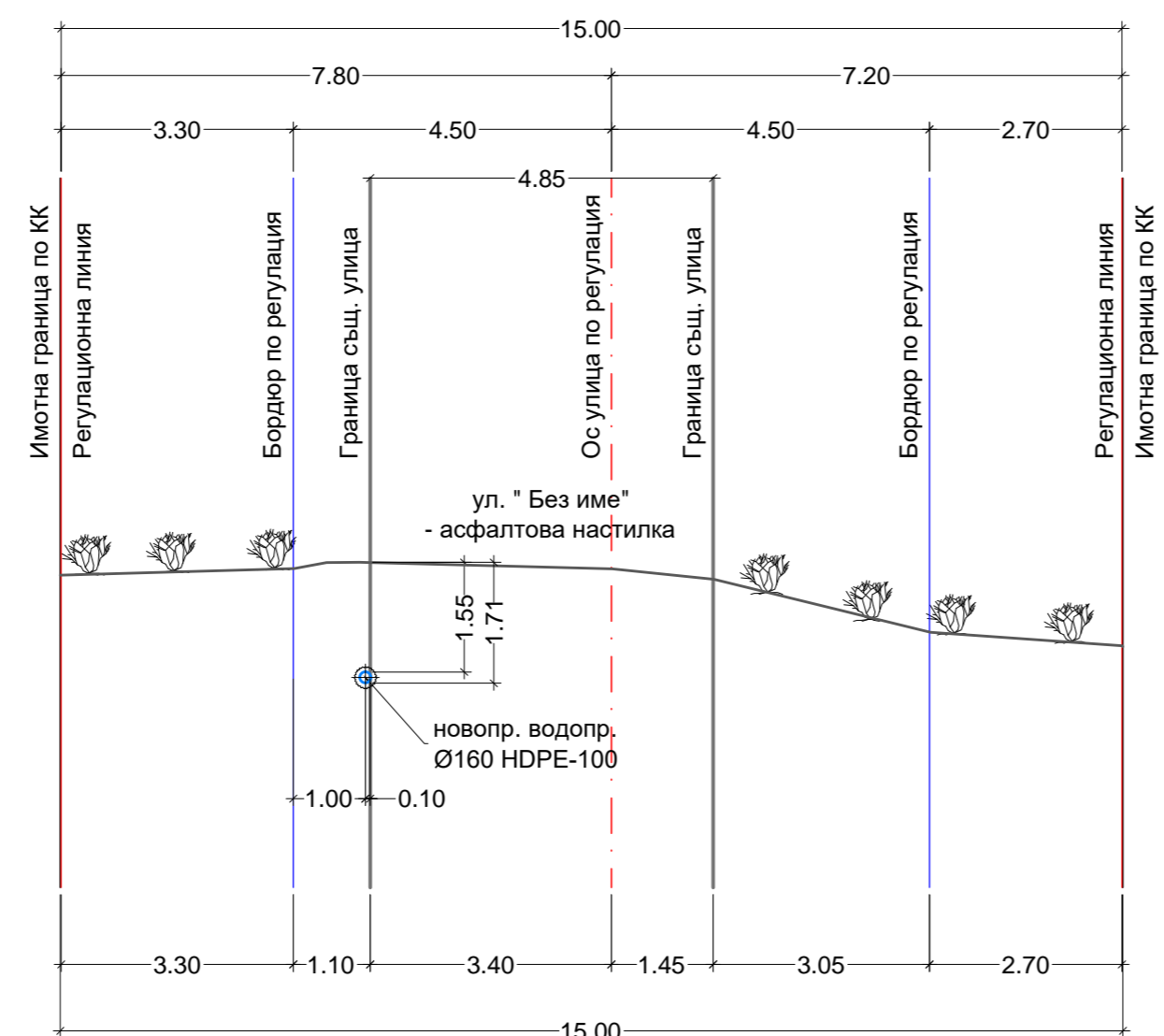
НАПРЕЧЕН РАЗРЕЗ №10 - хоризонтално сондиране
