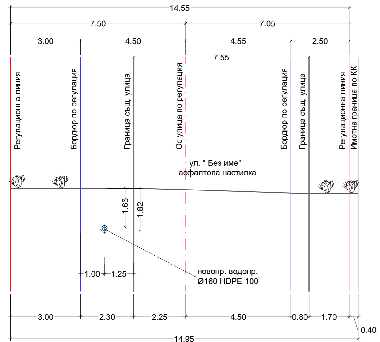
НАПРЕЧЕН РАЗРЕЗ №9 - открит вертикален изкоп
