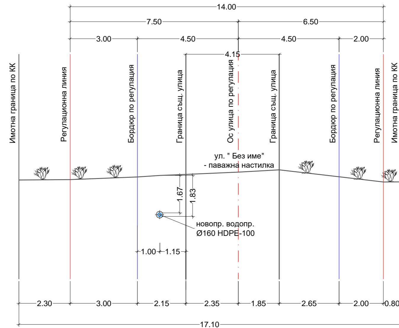
НАПРЕЧЕН РАЗРЕЗ №7 - хоризонтално сондиране
