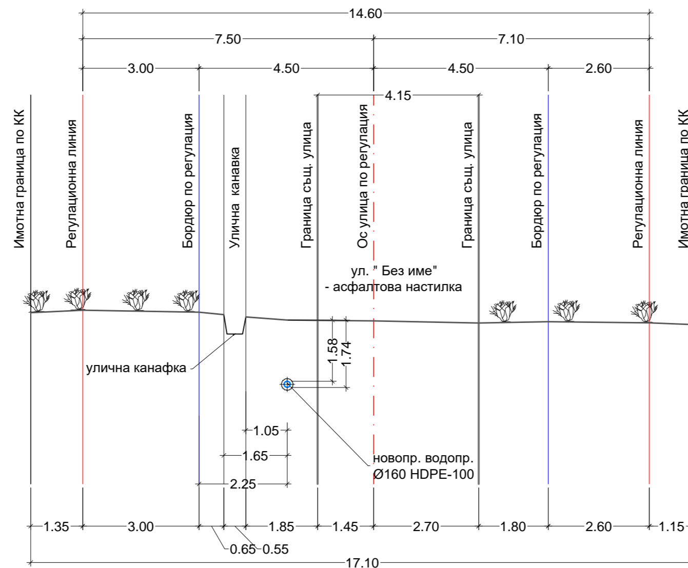
НАПРЕЧЕН РАЗРЕЗ №10 - хоризонтално сондиране
