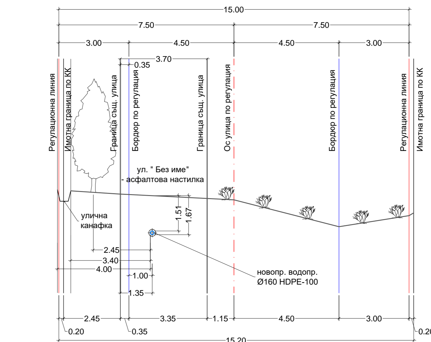
НАПРЕЧЕН РАЗРЕЗ №12 - хоризонтално сондиране
