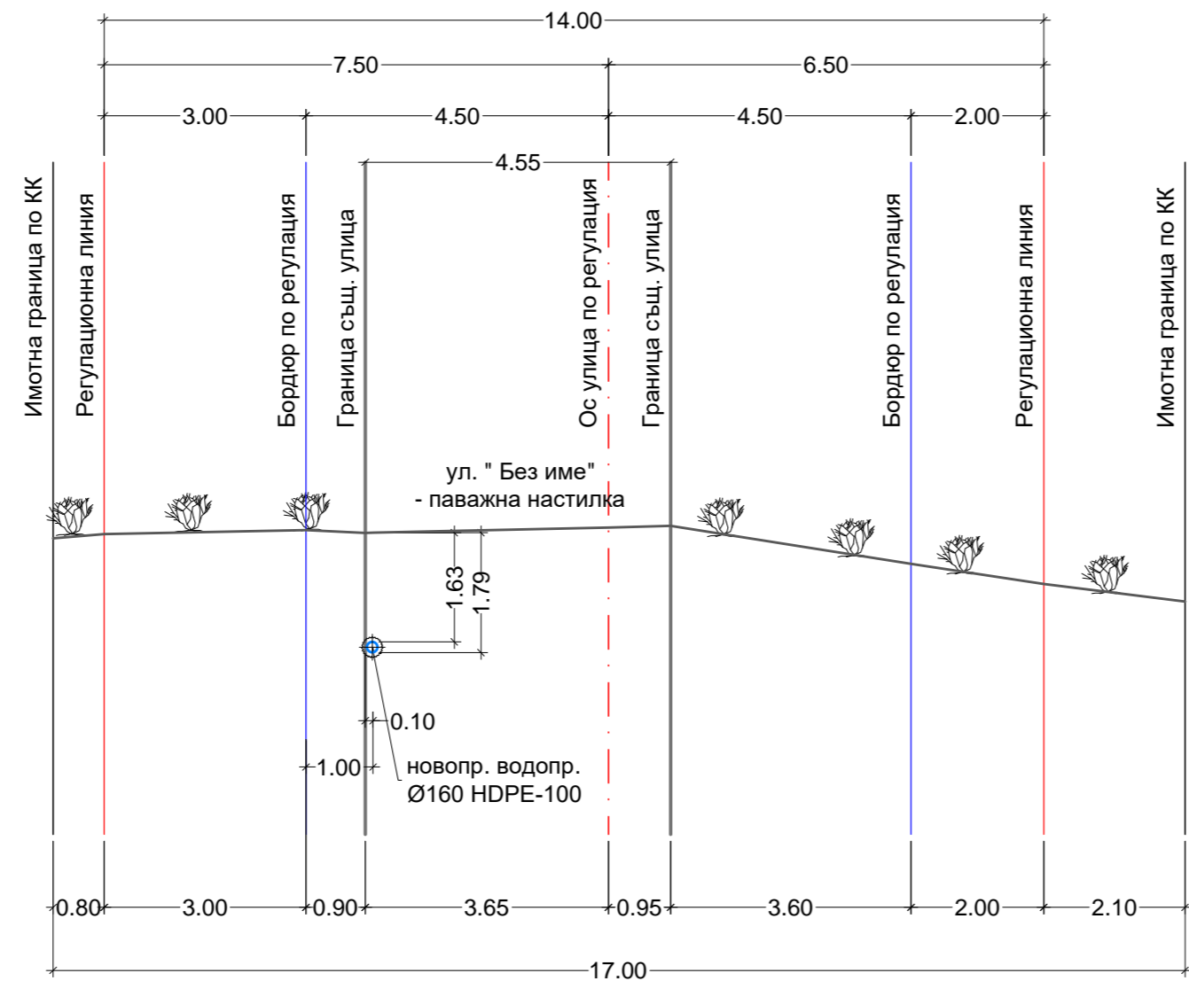
НАПРЕЧЕН РАЗРЕЗ №6 - хоризонтално сондиране
