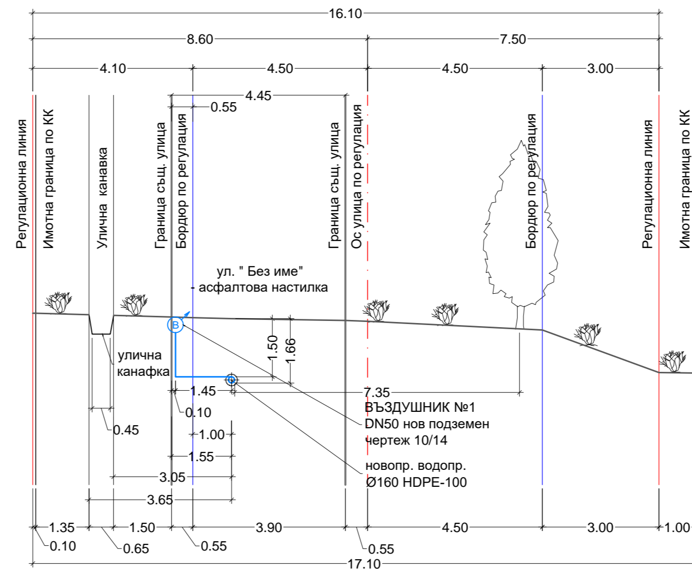
НАПРЕЧЕН РАЗРЕЗ №11 - хоризонтално сондиране
