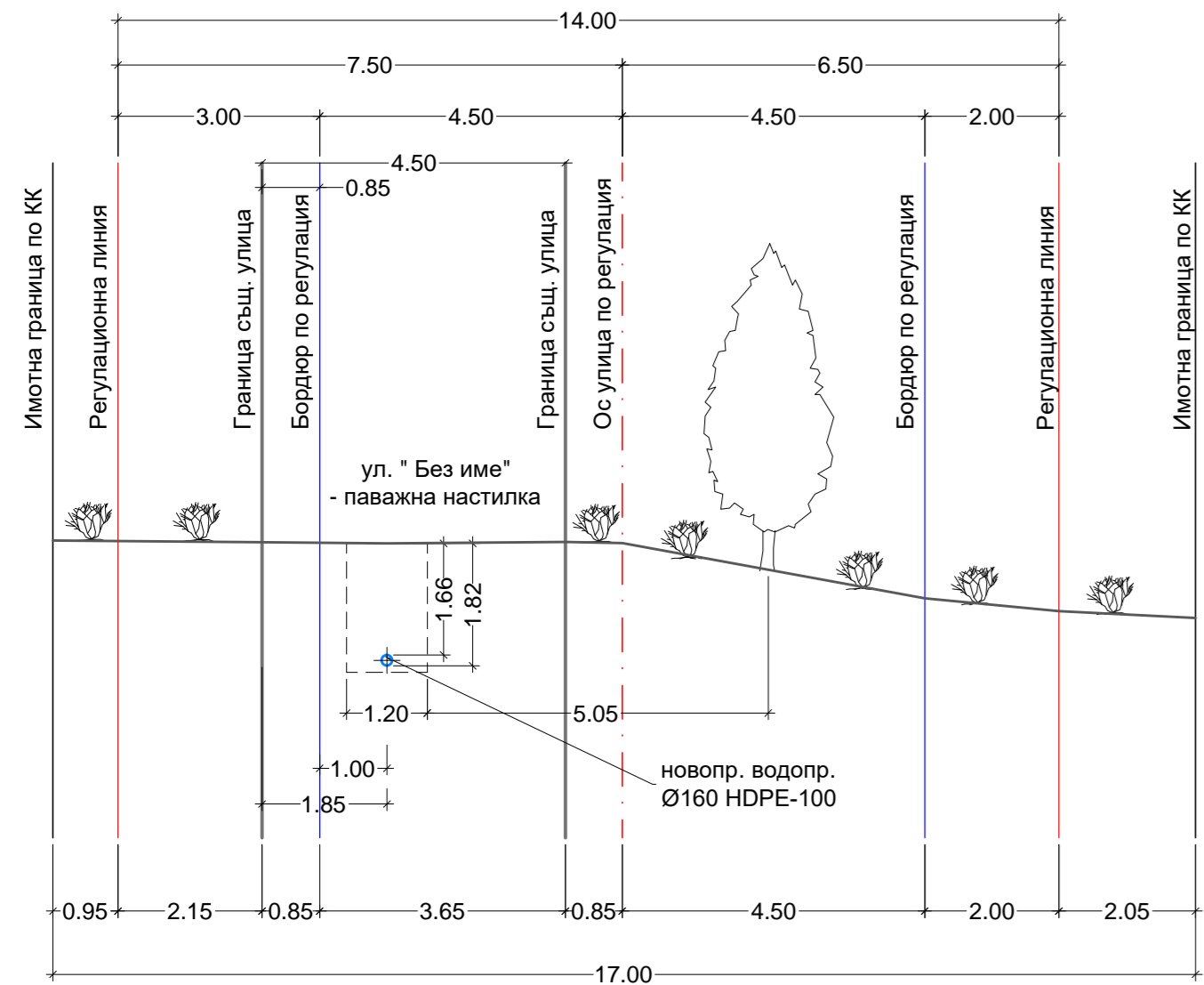
НАПРЕЧЕН РАЗРЕЗ №5 - хоризонтално сондиране
